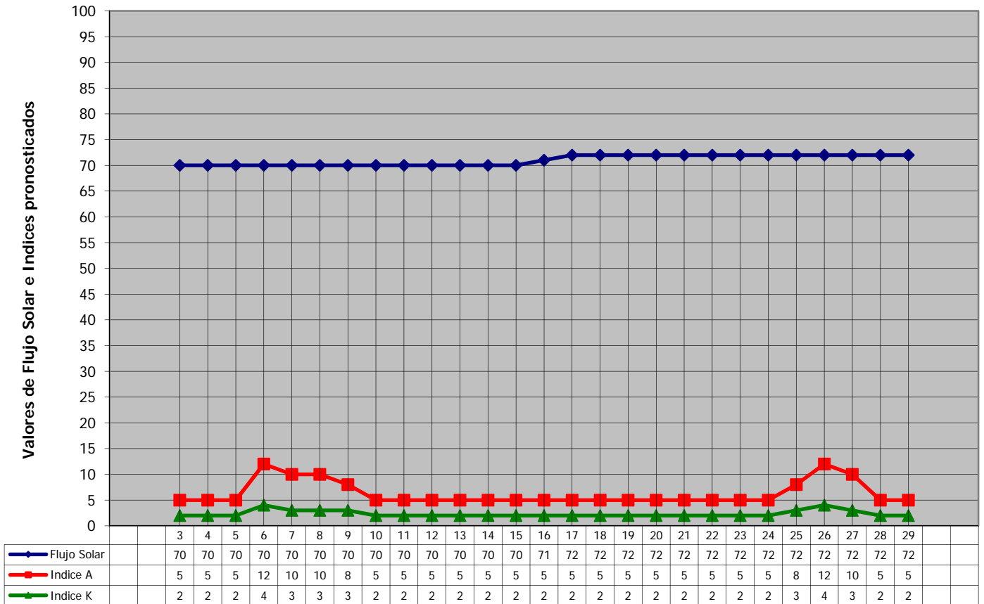
◆ Flujo Solar ■ Indice A ▲ Indice K Periodo Febrero 03 - Febrero 29 /2020
